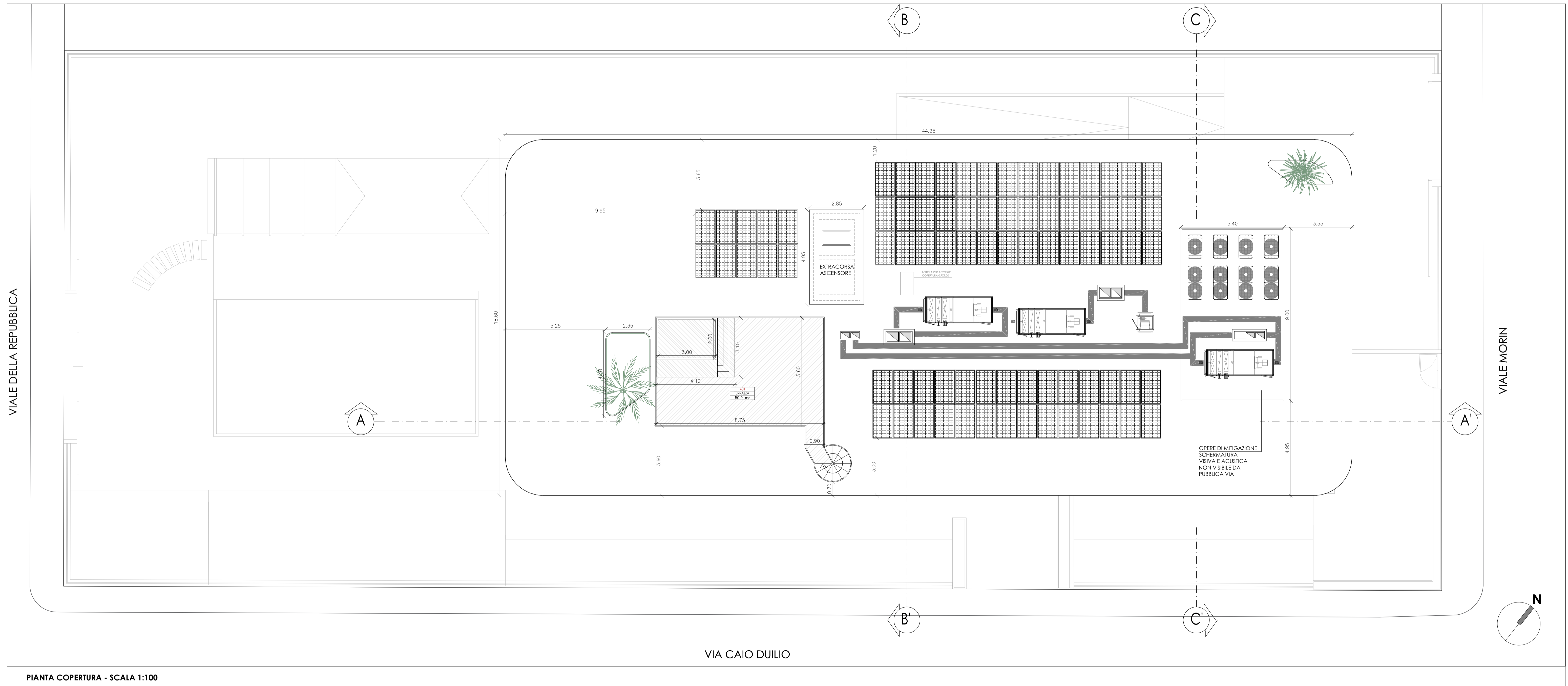
PIANTA COPERTURA - SCALA 1:100
