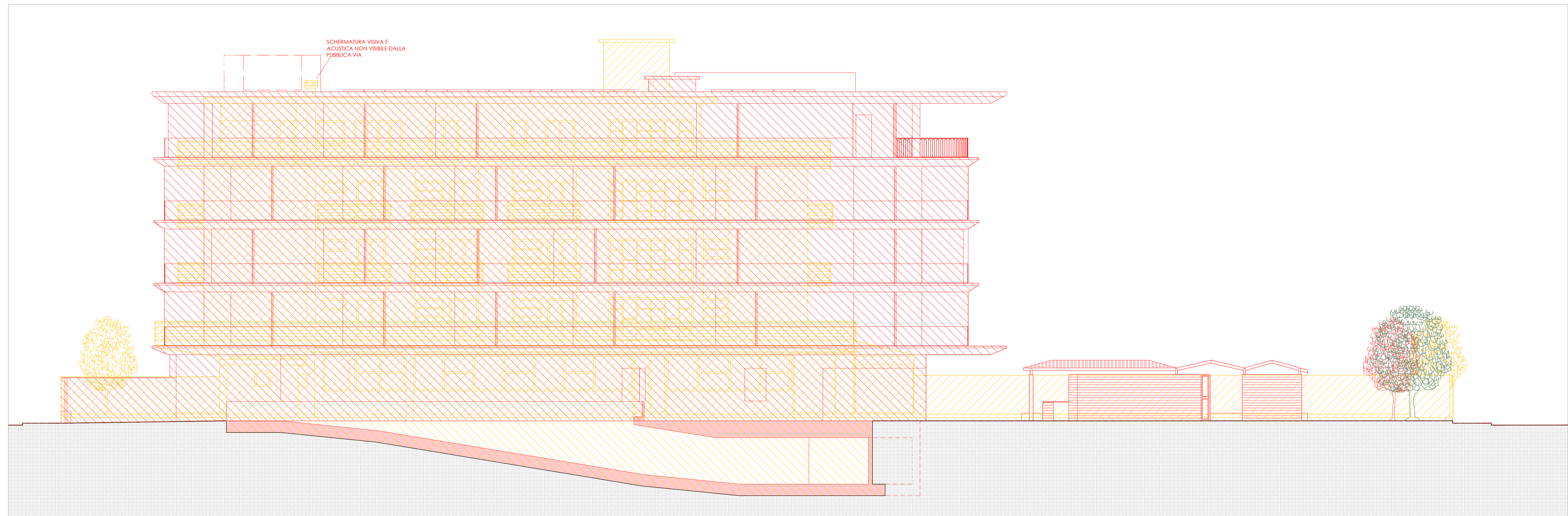
PROSPETTO 1 - NORD-OVEST 1:100
